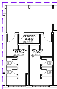
DET. PLANTA BAIXA ATUAL - W.C ALUNOS ESC. 1:75
