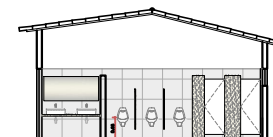
VISTA 01 BWC - MASC. ESC. 1:75
