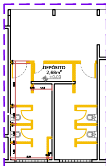
DET. PLANTA DE REFORMA - DEMOLIR - W.C ALUNOS ESC. 1:75
