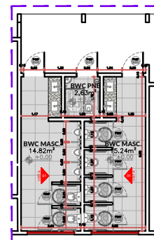
PLANTA BAIXA FINAL - W.C ALUNOS ESC. 1:75
