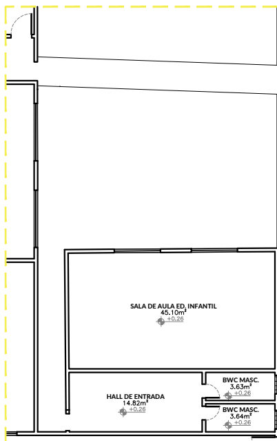
DET. PLANTA BAIXA FINAL - SALAS ED. INFANTIL ESC. 1:75
