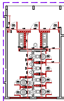
DET. PLANTA DE REFORMA - CONTRUIR - W.C ALUNOS ESC. 1:75
