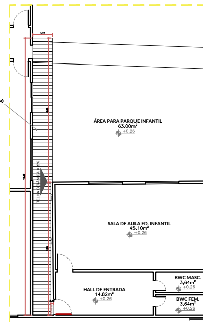
PLANTA DE COBERTURA - ACESSO SALAS ESC. 1:75
